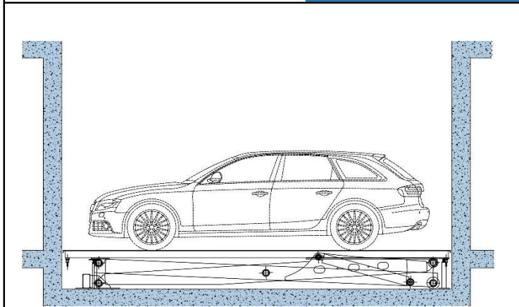
Vista in sezione -ALTO
