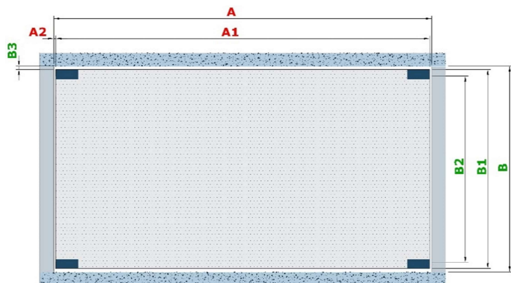
Dimensioni di ingombro
